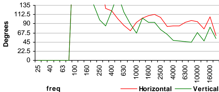
Beamwidth
