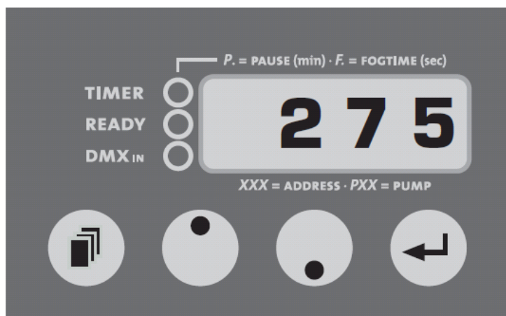
Obr. 2: Nastavení startovací adresy DMX
